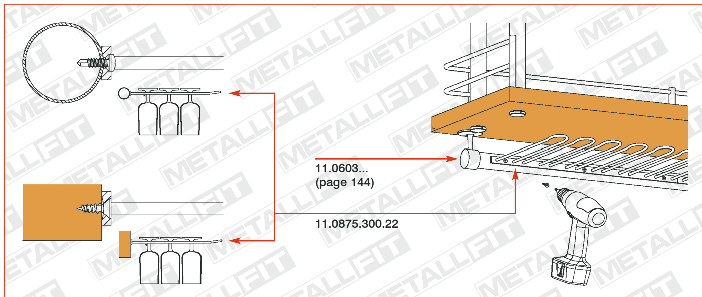
Glass rack Gläserhalter Ratelier à verres Glazenhouder
