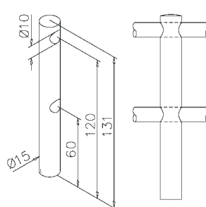
Double centre bracket / Doppelte Mittelstütze Support double traversant / Dubbele middensteun
