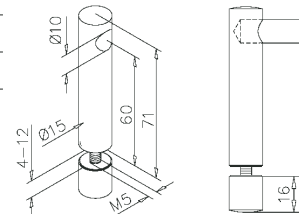
Centre bracket / Mittelstütze Support traversant / Middensteun
