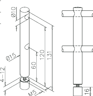
Double centre bracket / Doppelte Mittelstütze Support double traversant / Dubbele middensteun
