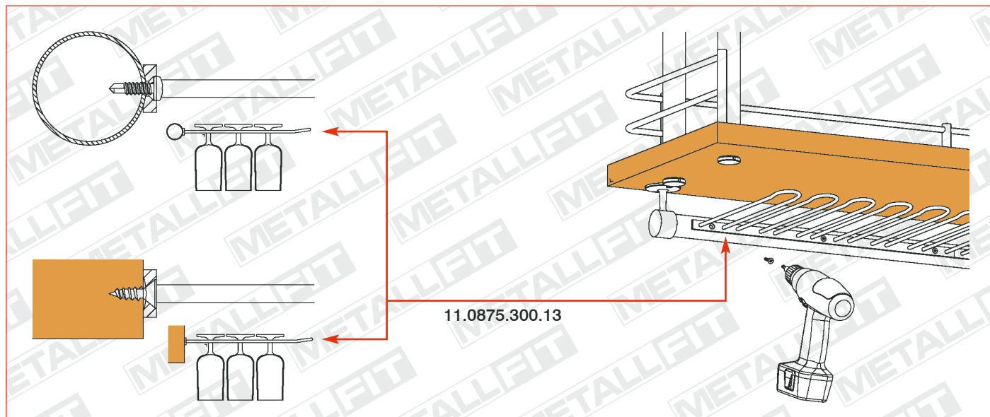
Glass rack Gläserhalter Ratelier à verres Glazenhouder
