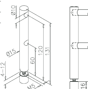
Double end bracket / Doppelte Endstütze Support double borgne / Dubbele eindsteun
