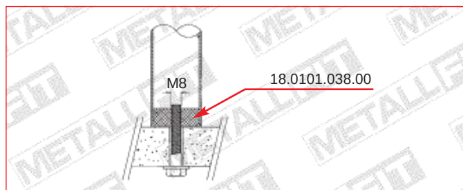
Nylon plug Kunststoff-Pfropfen Bouchon PVC taraudé Kunststof prop
