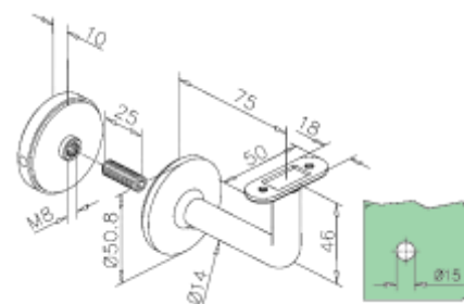
Flat handrail bracket for glass assembly, 8 - 12,76 mm Handlaufstütze flach für Glasmontage, 8 - 12,76 mm Support main-courante plate, fixation sur verre, 8 - 12,76 mm Vlakke leuninghouder voor montage op glas, 8 - 12,76 mm
