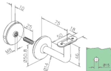
Flat handrail bracket for glass assembly, 8 - 12,76 mm Handlaufstütze flach für Glasmontage, 8 - 12,76 mm Support main-courante plate, fixation sur verre, 8 - 12,76 mm Vlakke leuninghouder voor montage op glas, 8 - 12,76 mm
