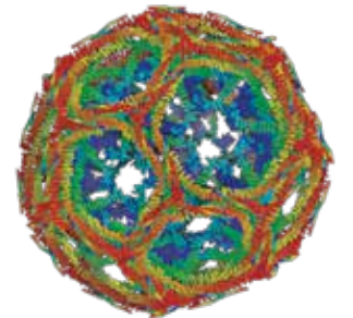
Clathrin
