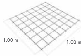
Malla electrosoldada de 4 mm 15 x 15 cm
